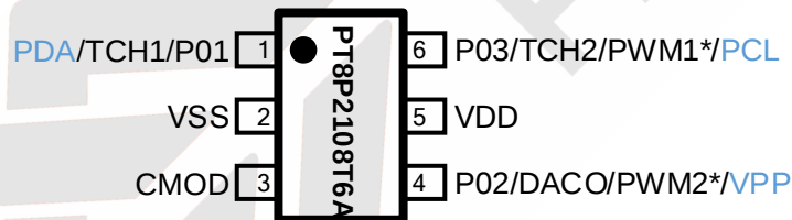
图 2 SOT23-6 封装示意图
