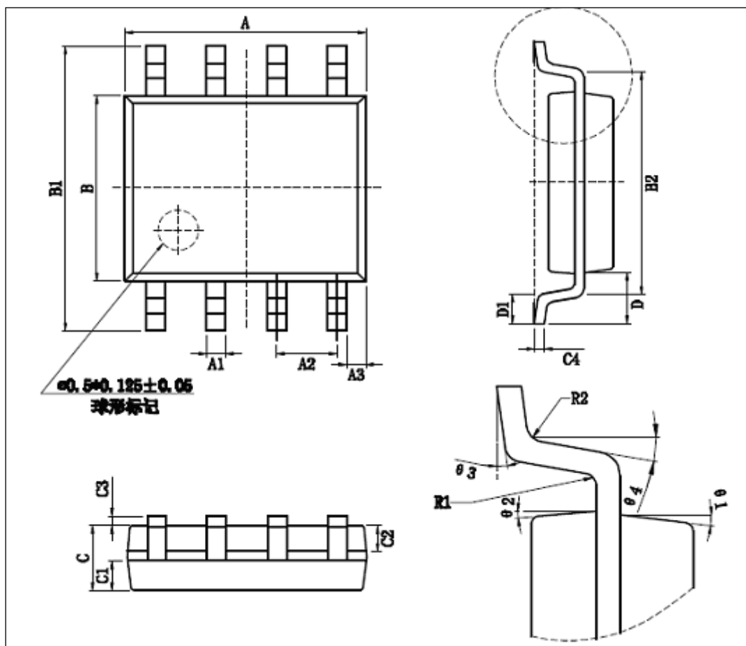
图 2 SOP8 封装
