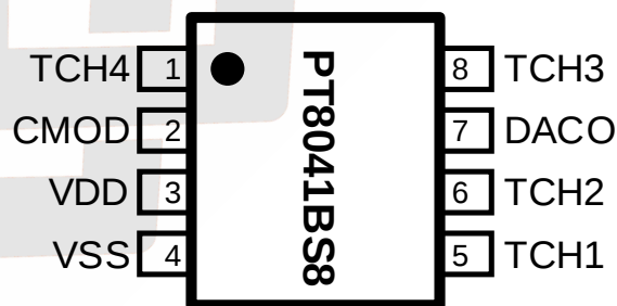
图 1 SOP8 管脚示意
